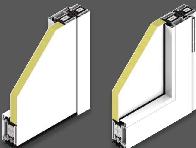
Außenansicht flügelüberdeckend
