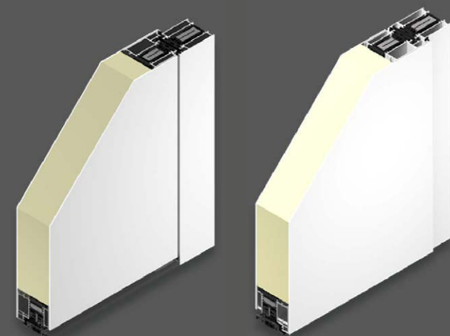
Außenansicht flügelüberdeckend
