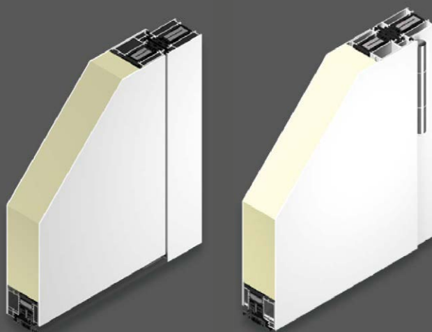
Außenansicht flügelüberdeckend
