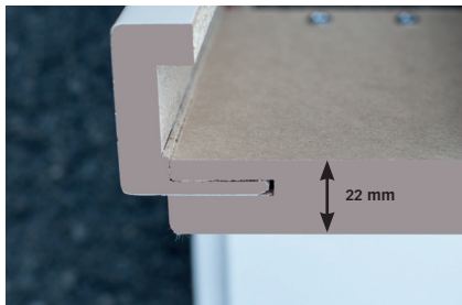
Stabilität der Herholz Zarge Geringe Verzugsanfälligkeit durch 22 mm Span-Futterplatte
