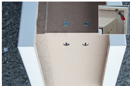
Patentierter GMF-Verbindung Perfekte Montageergebnisse der Gehrung durch die patentierte GMF-Verbindung mit kraftschlüssiger Verschraubung
