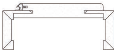
Furnierte Softzarge FR 60 mm Bekleidung abgerundet R2, ohne Profil Bekleidungen auf Gehrung
