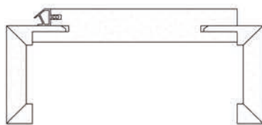
G65 Normzarge eckig 65 mm Bekleidung eckig, ohne Profil Bekleidungen auf Gehrung
