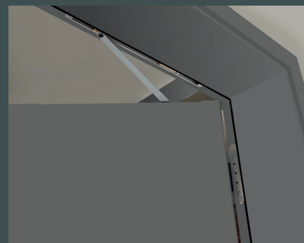
Obentürschließer (OTS) (Gleitschienen-Türschließer optional)
